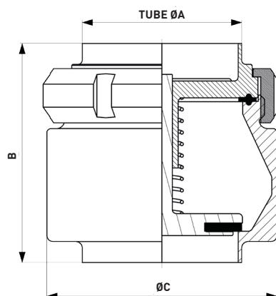
CLAPET ANTI-RETOUR SORTIE TUBE
